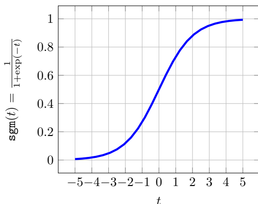
sigmoid function
